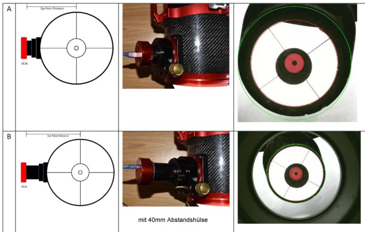
Abb. 3.1: Fokuslage
